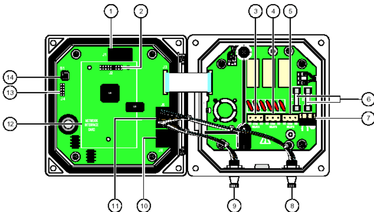
图 15 布线连接
